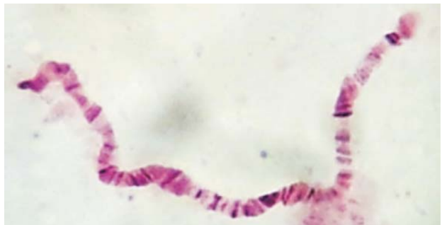
Fig. 7. Chromosome 5 (3L)
