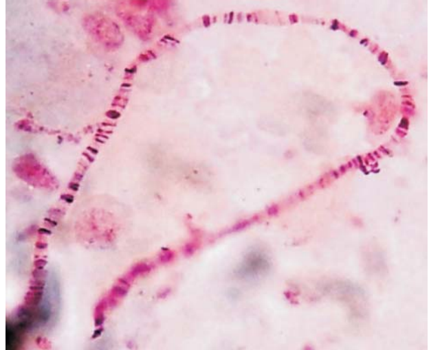
Fig. 4. Chromosome 2 (2R)
