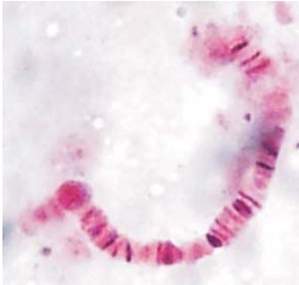
Fig. 3. Chromosome X
